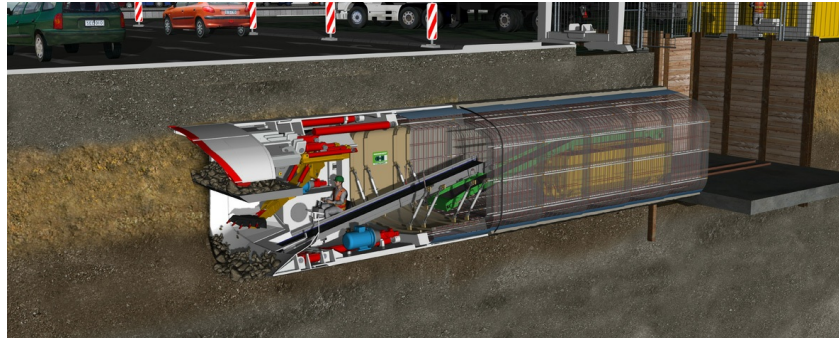
Ausbauvariante mit Ortbeton direkt hinter der Maschine.
